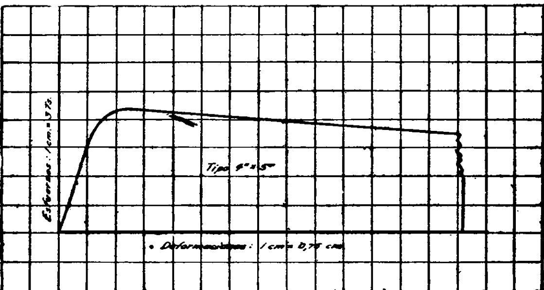
Gráfico N.º 4. Ensayo de una pieza de ROBLE PELLIN
